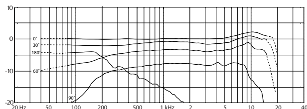
典型的轴向和离轴响应, 4099 在 20 cm 距离处
