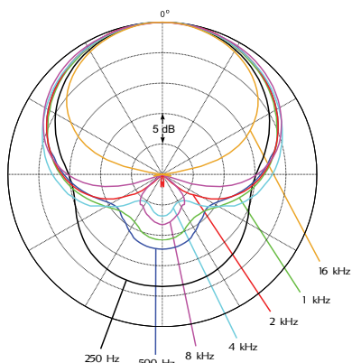
4099的指向性 (规格化)
