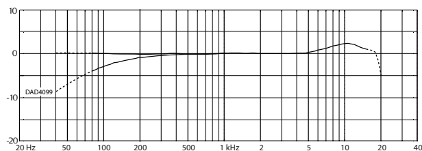
典型频率响应, 4099使用DAD4099卡侬连接器, 在20 cm (7.9 in) 厘米处
